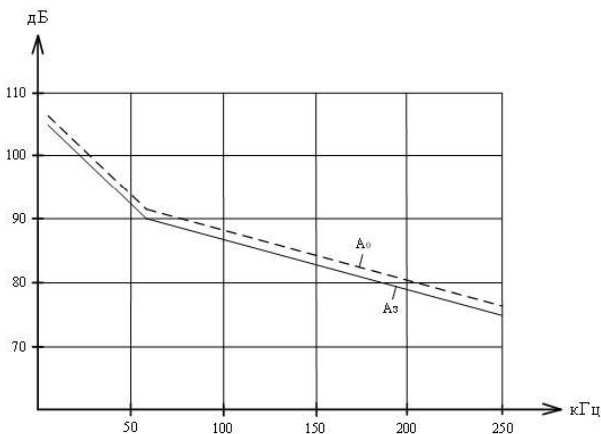
Рисунок 2. Частотные характеристики переходного затухания на ближнем конце A_0 и защищенности на дальнем конце A_z (усредненные значения) кабеля СБМВБАБпШп 19х2х1,0
